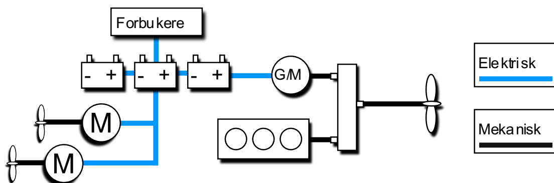
Figur 2: Prinsippskisse, parallell-hybridløsning
